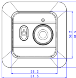
Внешняя рамка
