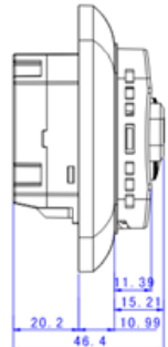
Габариты
